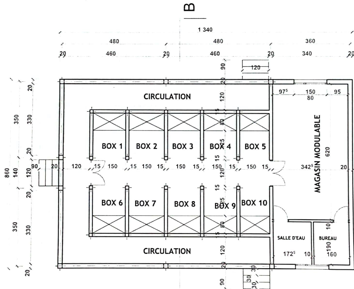
B PLAN DE DISTRIBUTION
